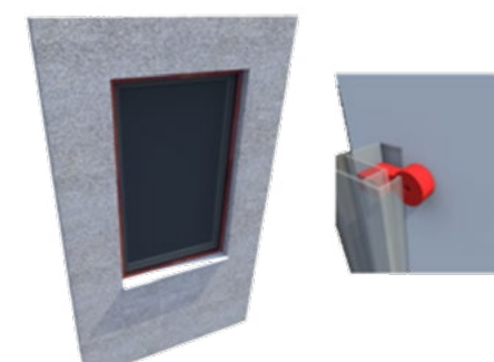
Végül fordítsa el 90°-kal a rögzítő elemeket
