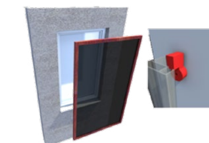
Majd helyezze fel a fix szúnyogháló keretét az ablakkeretre
