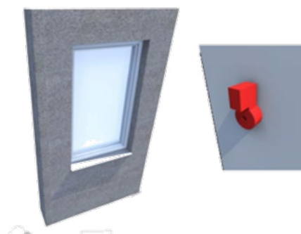
Csavarozza fel a rögzítő elemeket az ablakkeretre
